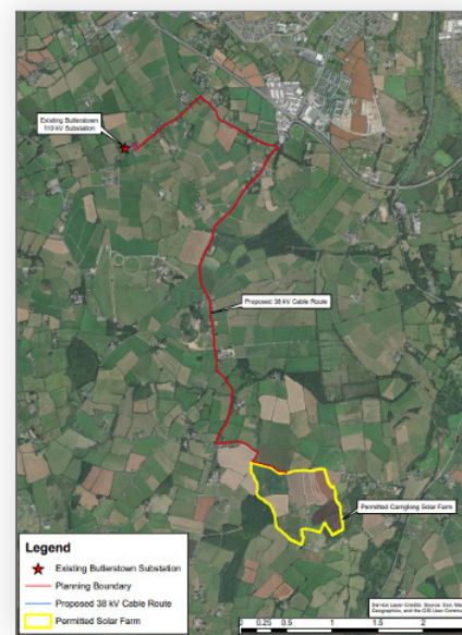
Fóir 2 Slí an chábla faoi thalamh
